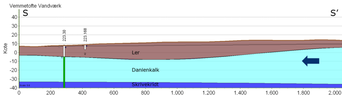
Figur B1.71: Geologisk profil gennem indvindingsoplandet til Vemmetofte Kloster Vandværk.
