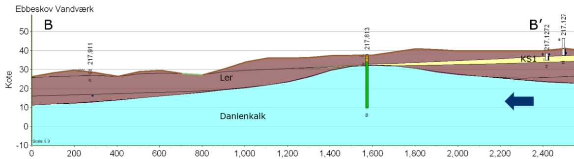
Figur B1.6: Geologisk profil gennem indvindingsoplandet til Ebbeskov Vandværk.
