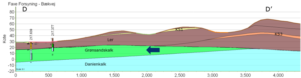
Figur B1.14: Geologisk profil gennem indvindingsoplandet til Faxe Forsyning, Haslev, Bækvej Vandværk.
