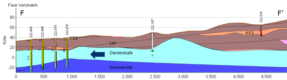
Figur B1.22: Geologisk profil gennem indvindingsoplandet til Faxe Vandværk.
