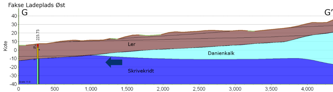
Figur B1.26: Geologisk profil gennem det østlige indvindingsopland til Fakse Ladeplads Vandværk.
