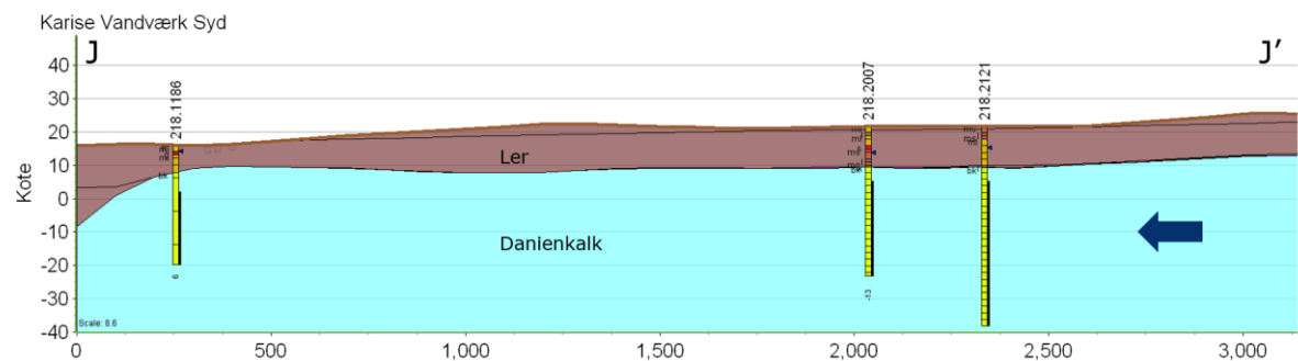
Figur B1.32: Geologisk profil gennem det nordlige indvindingsopland til Karise Vandværk.
