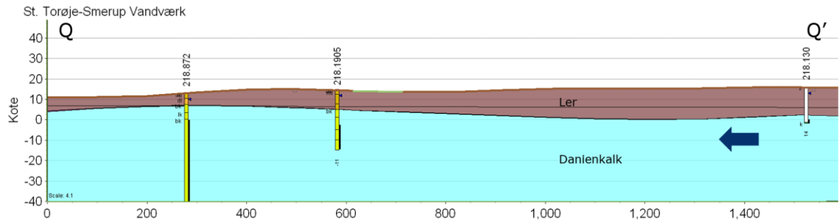
Figur B1.63: Geologisk profil gennem indvindingsoplandet til St. Torøje-Smerup Vandværk.
