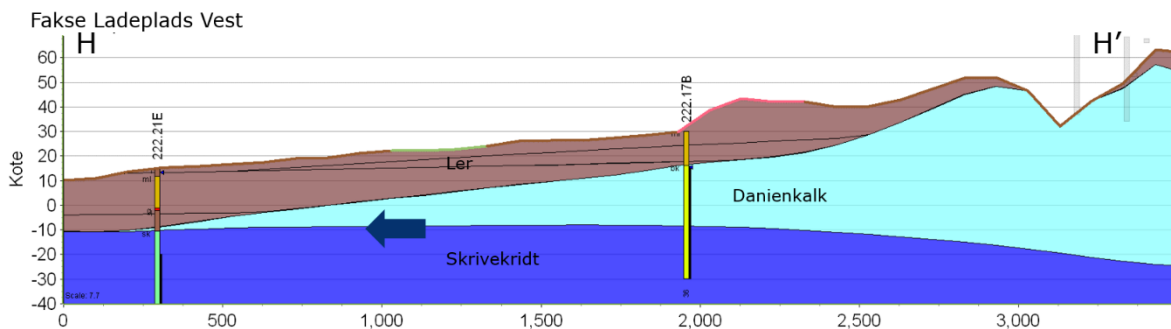
Figur B1.27: Geologisk profil gennem det vestlige indvindingsopland til Fakse Ladeplads Vandværk.
