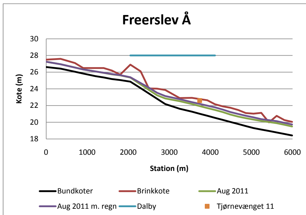
Figur 3-4 Modellerede vandstandsforhold i Freerslev Å, langs Dalby. Bundkoten er gengivet med sort, terræn med rød, udstrækningen af byen med lyseblå og terrænkoten ved Tjørnevænget 11 med orange markering.
