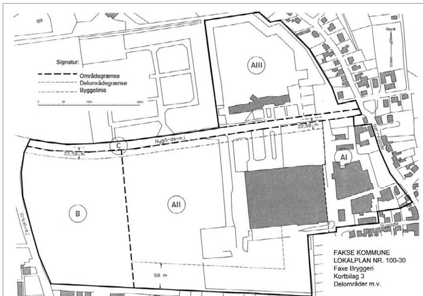
Flyfoto set mod nord (jan. 2007) med det store bryggerikompleks mellem Nørregade og Faxe Allé. Til venstre Faxe Industripark. Herunder lokalplan nr. 100-30, fra 1997 med bryggeriets forskellige byggelinier og arealudlæg. AI er produktions- og tappehaller, mens AIII er administration. B er reserveareal.
