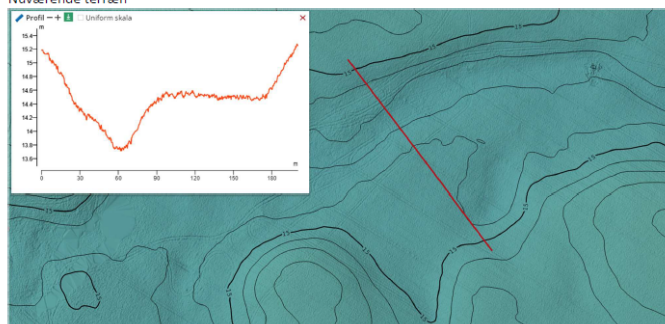
Tværsnit 1:
