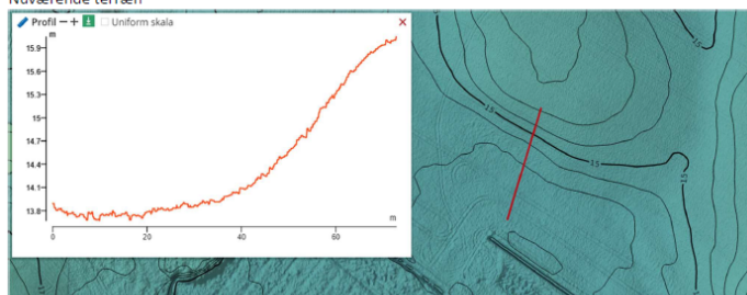
Tværsnit 3:
