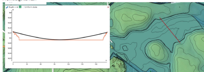
Tværsnit 3:
