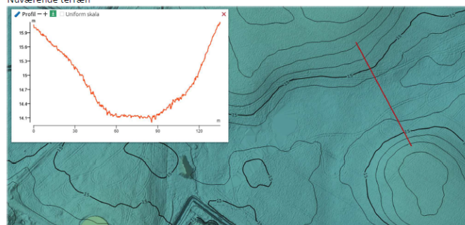
Tværsnit 2:
