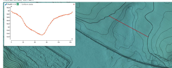
Tværsnit 4:
