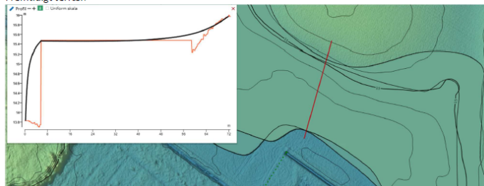
Tværsnit 5:
