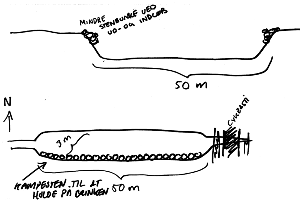
Figur 4: Skitsetegning over sandfangets udformning.
